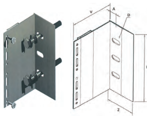
STAFFA LUNGA
