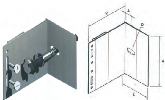
STAFFA NORMALE
